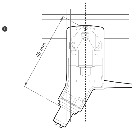
① カートリッジの針先
