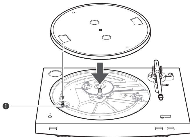
① モータープーリー（金色）
