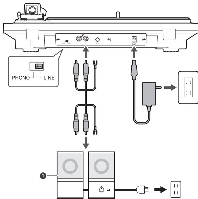
❶ 主動式揚聲器
