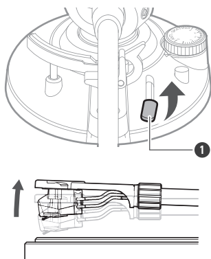
① リフターレバー
