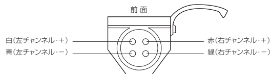
前から見たシェルリード線の配列(ユニバーサルアームの場合)
