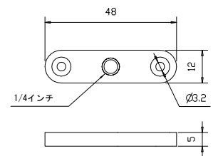
カメラネジアダプター
