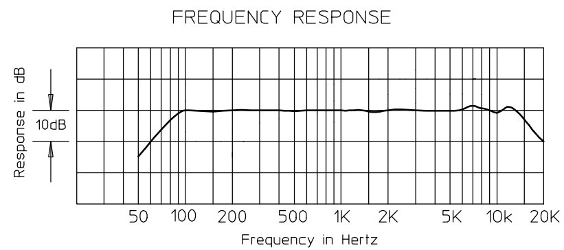
周波数特性
