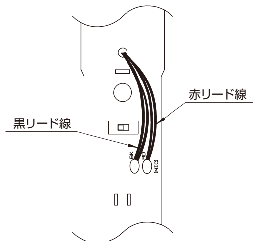
図1. PCB裏面 (TX)
